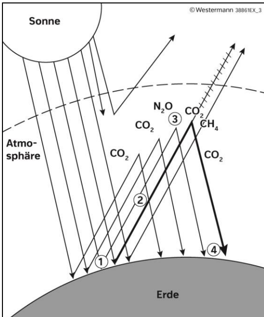
M1 Der natürliche Treibhauseffekt
