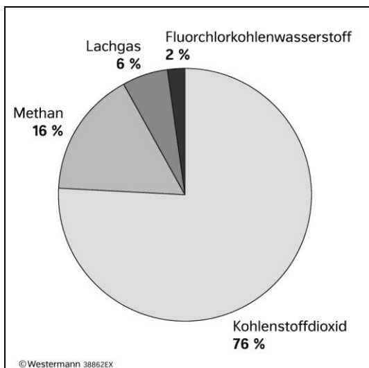
M2 Wirkungsanteil der Gase am Treibhauseffekt
